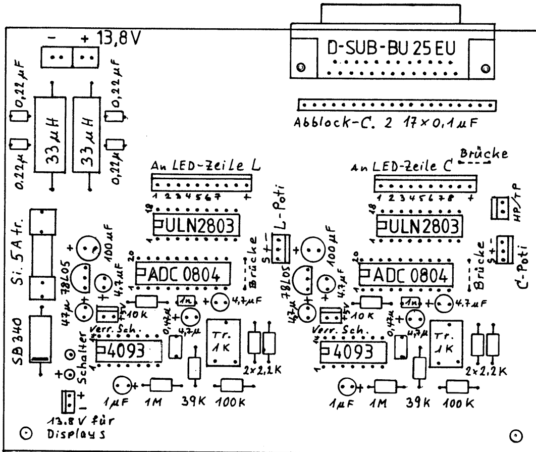
Bestückungsplan Steuerplatine
