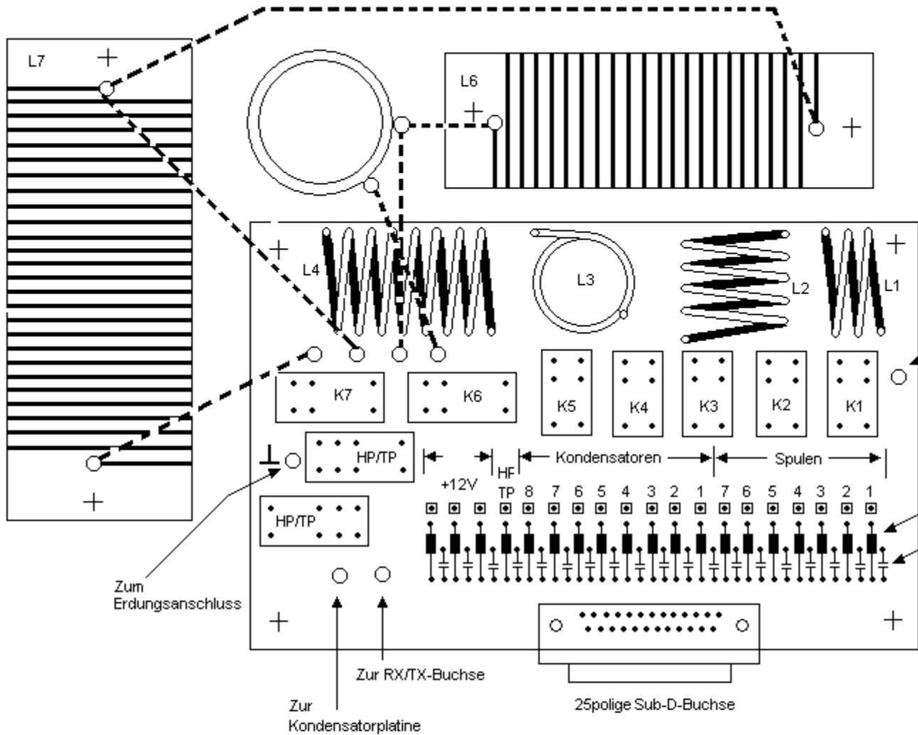
Christian-Langdrahtkoppler Bestückungsplan Spulenplatine Maßstab etwas größer als 1:1
